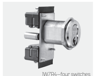
1W7R4—four switches
